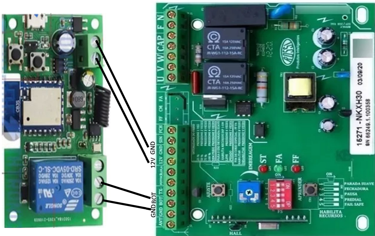
Conexão em Motor de Portão
